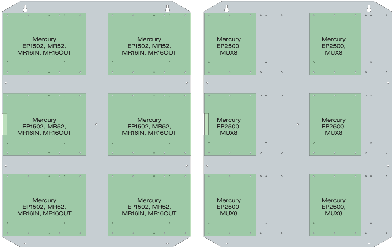
TMV2 - Optional Door Backplane Configurations:
